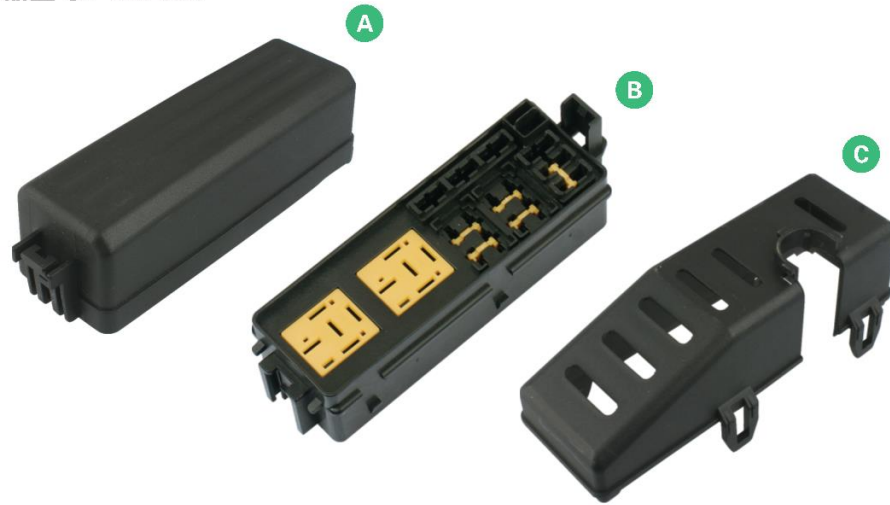
产品名称：6路保险盒总成 产品型号：BX2061
