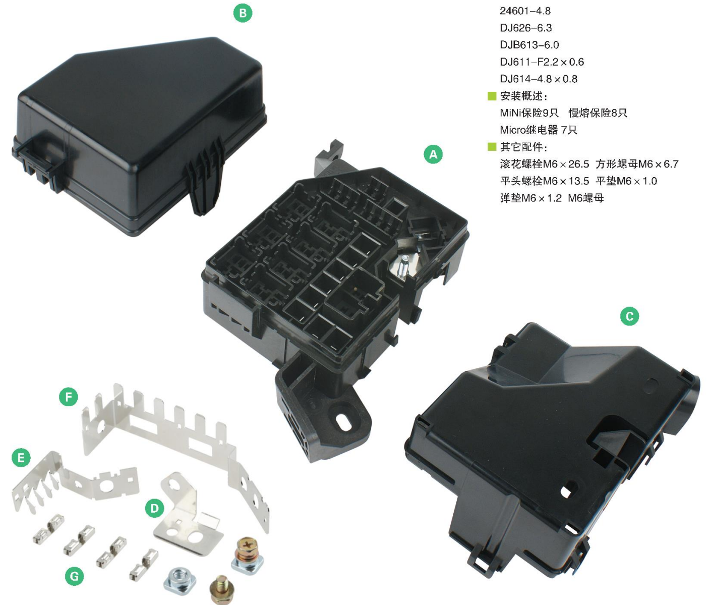
产品名称：9路保险盒总成 产品型号：3724111
